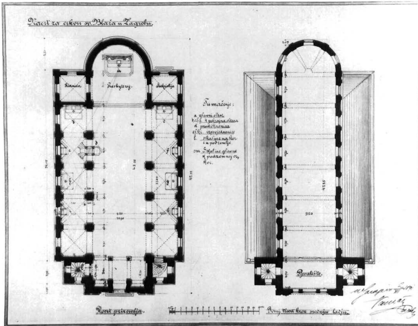
Josip Vančaš, tlocrt prizemlja i gornji tlocrt srednjega broda, 2. 12. 1891. (KAZ; foto: I. Buzjak)
