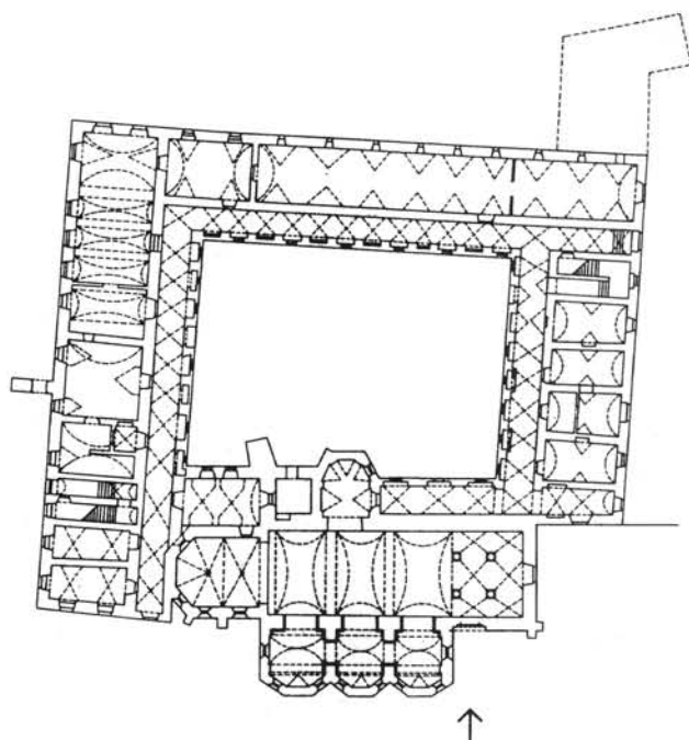
Tlocrt crkve i samostana s položajem sjevernog portala (prema arh. snimci M. Puncera)
