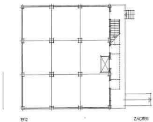
Aladar Baranyai: Zgrada trgovačke tvrtke Socher u Preradovićevoj ulici, 1912. Tlocrt i presjek prema urudžbenom planu, precrt arhivske građe: A.L.
